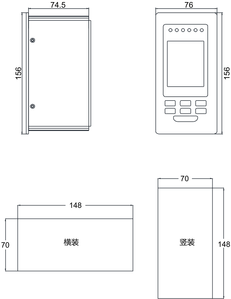
开孔尺寸
